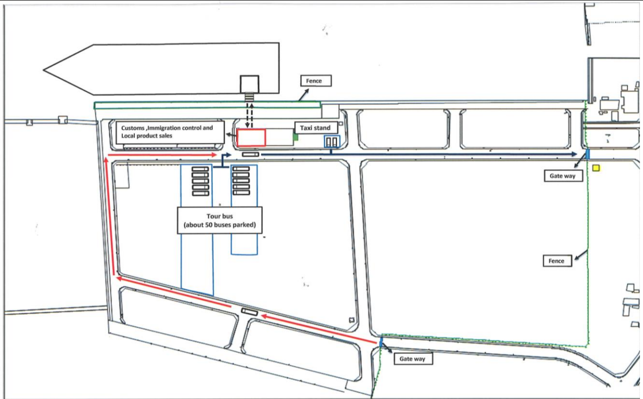
ターミナル配置図と受入動線
